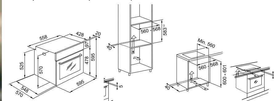
Схема установки для духовых шкафов Maris
